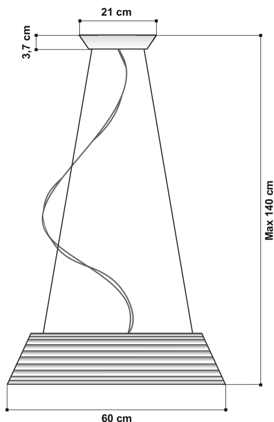
Dimensioni - Dimensions
