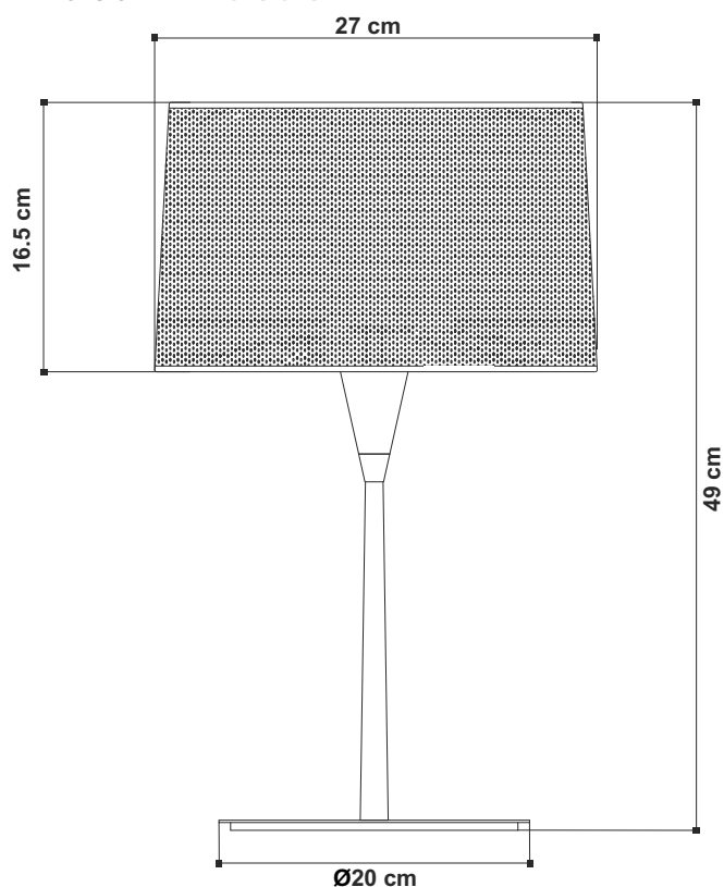
Dimensioni - Dimensions
